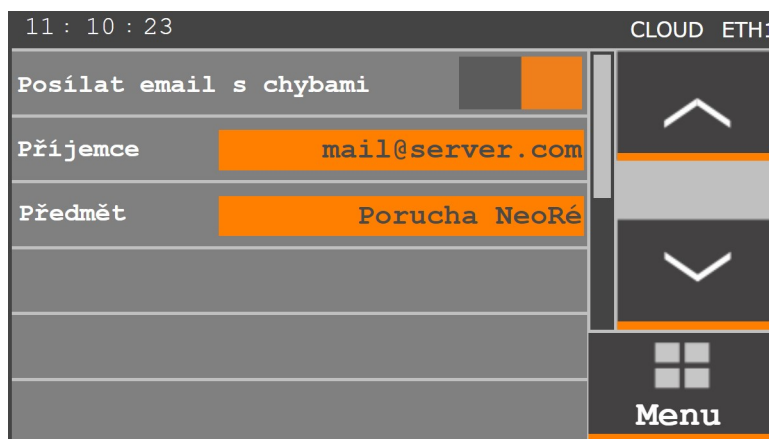
Obrázek 4.27: Sekce nastavení - obrazovka 2 → Nastavení sítě 1 → Nastavení e-mailu
