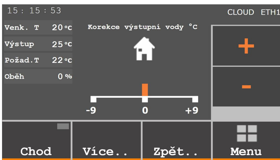
Obrázek 2: Základní obrazovka SIMPLE NEO pro korekci ekvitermní křivky
