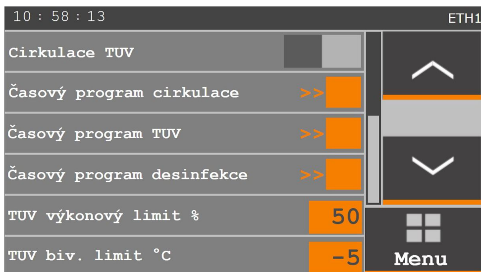
Obrázek 4.19: Sekce TUV - obrazovka 2
