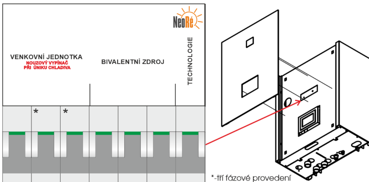
Obrázek 5.1: Jistící prvky tepelného čerpadla
