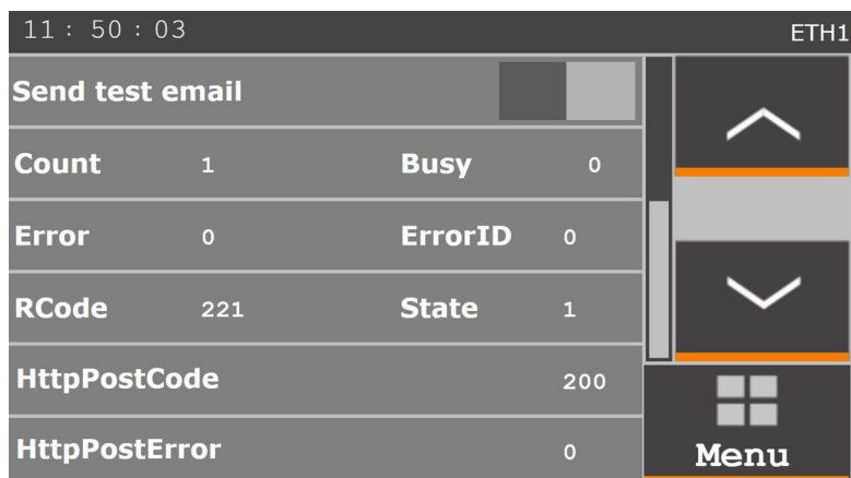
Obrázek 4.28: Sekce nastavení - obrazovka 2 → Nastavení sítě 3 → Statistika e-mailu
