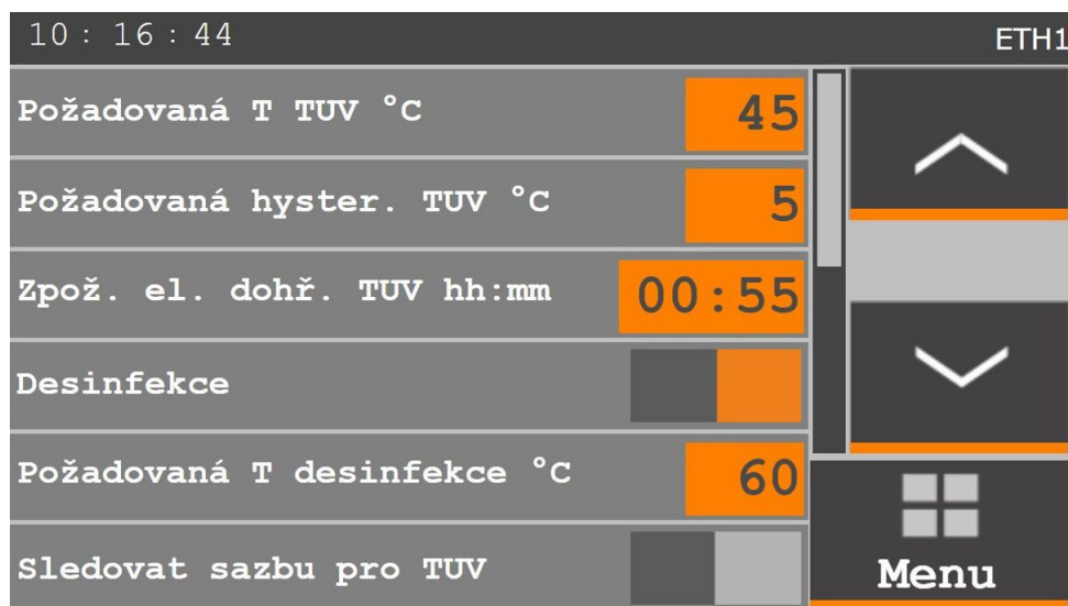
Obrázek 4.18: Sekce TUV - obrazovka 1
