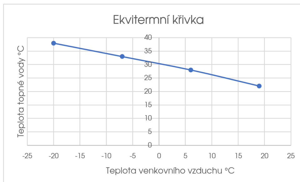
Obrázek 4.14: Graf - Ekvitermní křivka
