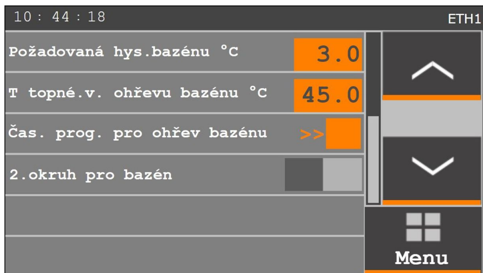
Obrázek 4.35: Sekce Další - obrazovka 2
