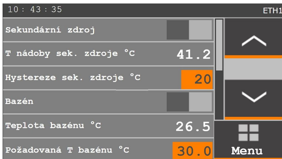
Obrázek 4.34: Sekce Další - obrazovka 1
