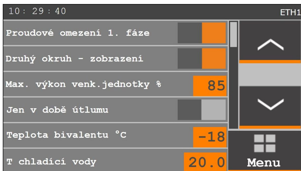
Obrázek 4.22: Sekce nastavení - obrazovka 1
