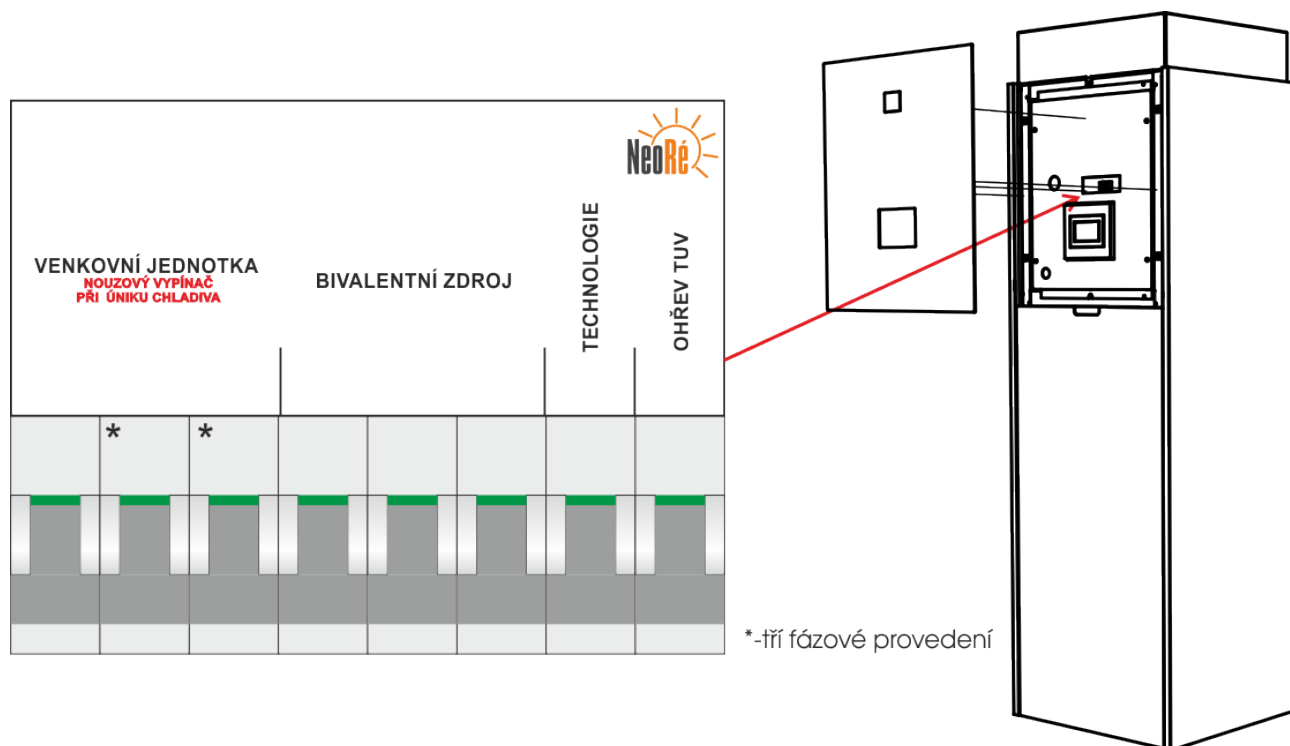
Obrázek 5.1: Jisticí prvky tepelného čerpadla
