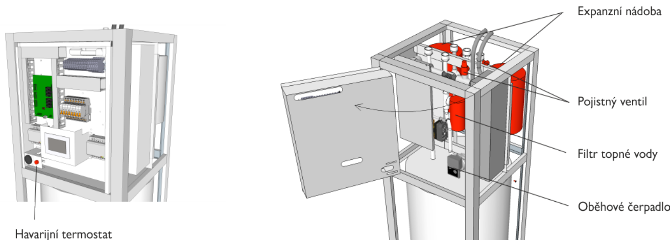
Obrázek 8.1: Základní popis vnitřní jednotky
