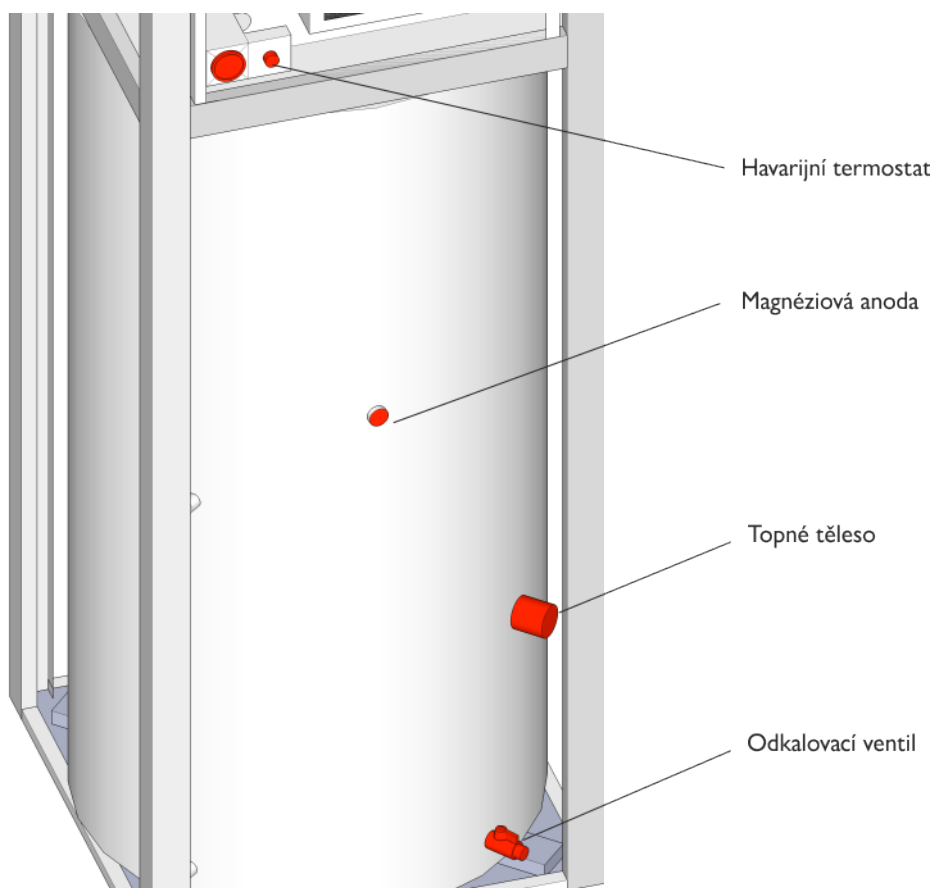
Obrázek 8.2: Popis zásobníku TUV
